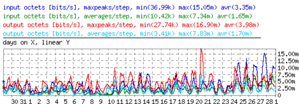
obrázek 3: PRŮMĚRNÝ PROVOZ V ÚNORU 2003 Z CESNETU Z/DO JINDŘICHOVA HRADCE (PŘEVZATÁ STATISTIKA CESNETU)
