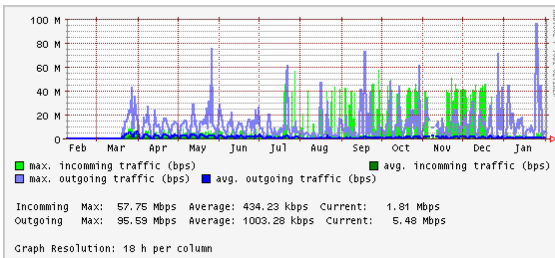
Obrázek 2: Průměrný provoz od března roku 2004 z areálu na Jižním Městě do/z PASNETu
